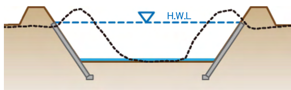
図-4.5 早川 代表横断面
