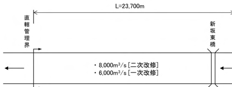
図-4.3 計画流量配分図
