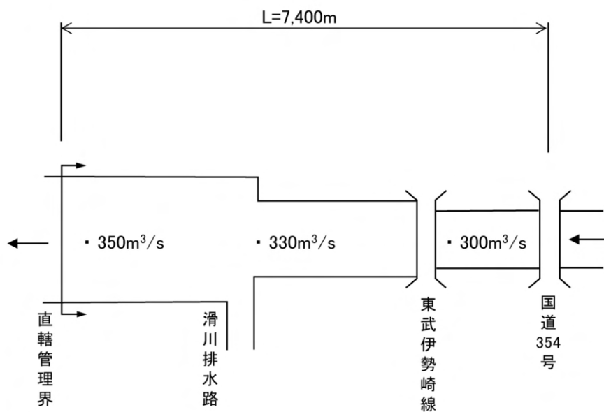
図-4.6 計画流量配分図
