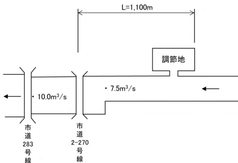
図-4.9 計画流量配分図
