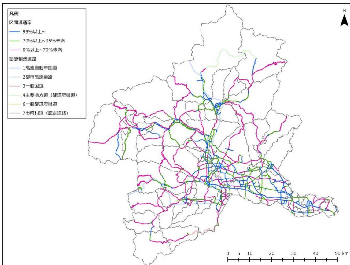
図 3-4-21 2 地点間の導通率（深谷断層帯・綾瀬川断層、夏 12 時、強風）
