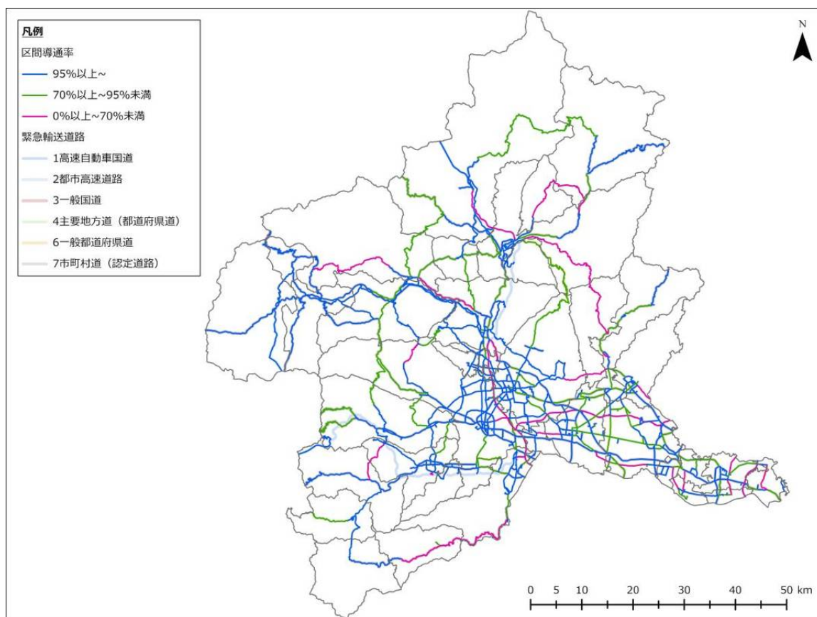
図 3-4-22 2 地点間の導通率（太田断層、冬 18 時、強風）
