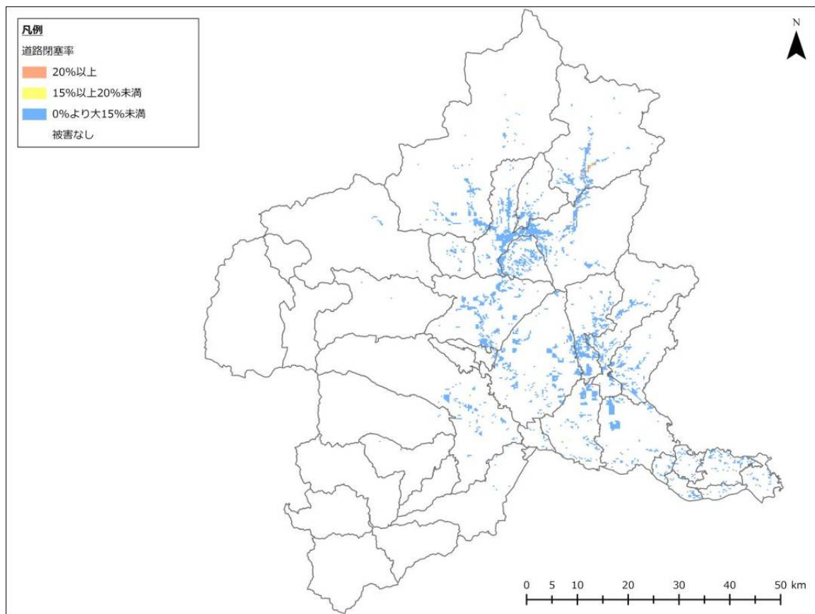
図 3-4-9 道路閉塞率（片品川左岸断層、夏 12 時、強風）
