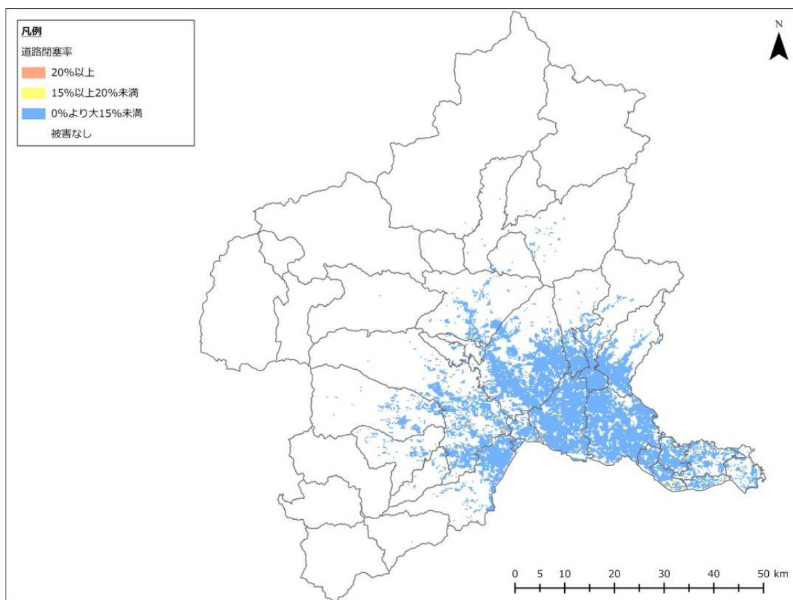
図 3-4-5 道路閉塞率（太田断層、冬 5 時、強風）
