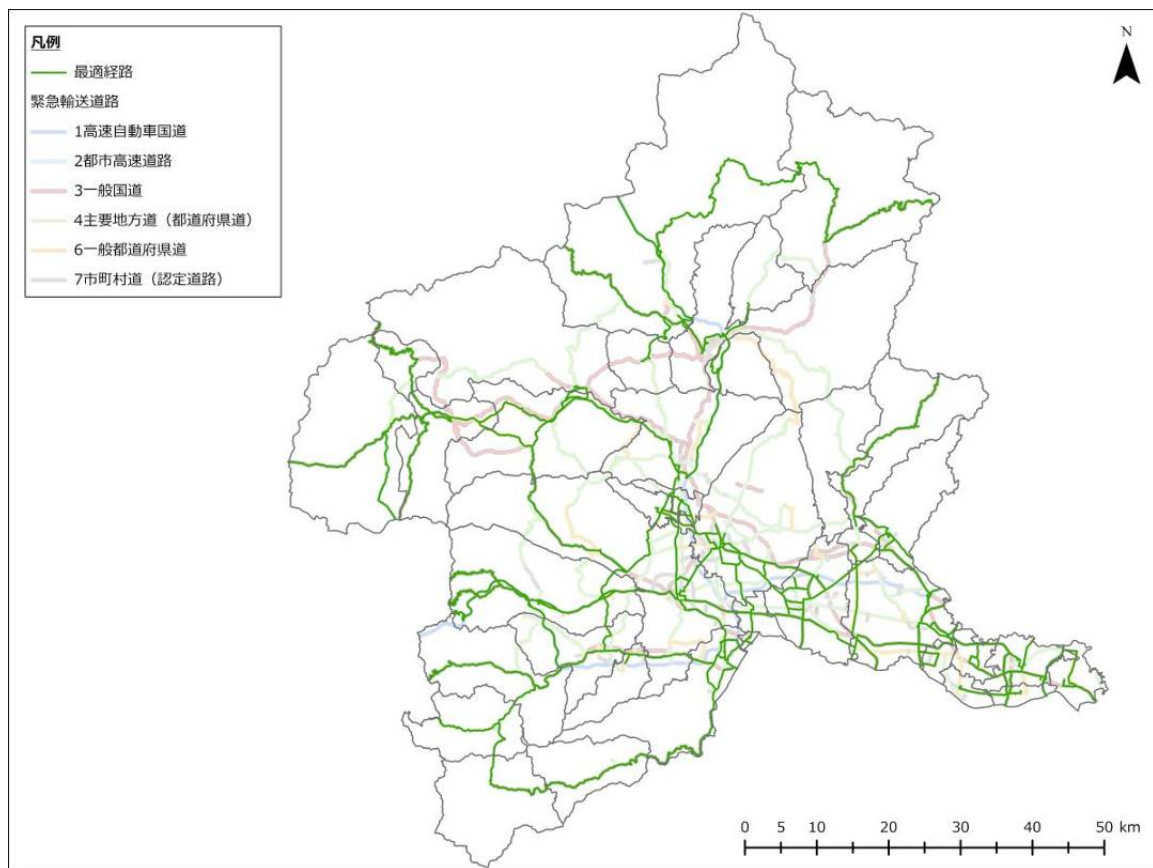
図 3-4-45 主要都市間の最適経路（片品川左岸断層、夏 12 時、強風）
