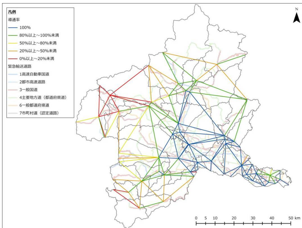
図 3-4-71 主要都市間の導通率（長野盆地西縁断層帯、冬 5 時、強風）
