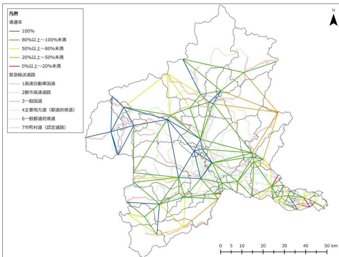
図 3-4-59 主要都市間の導通率（太田断層、冬 5 時、強風）
