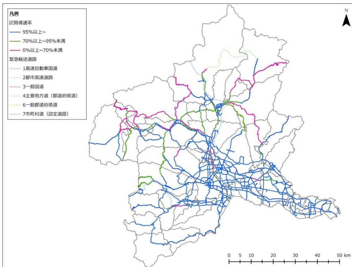
図 3-4-31 2 地点間の導通率（六日町断層帯、冬 18 時、強風）
