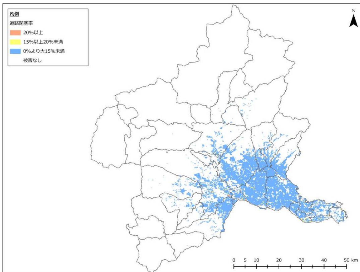
図 3-4-6 道路閉塞率（太田断層、夏 12 時、強風）
