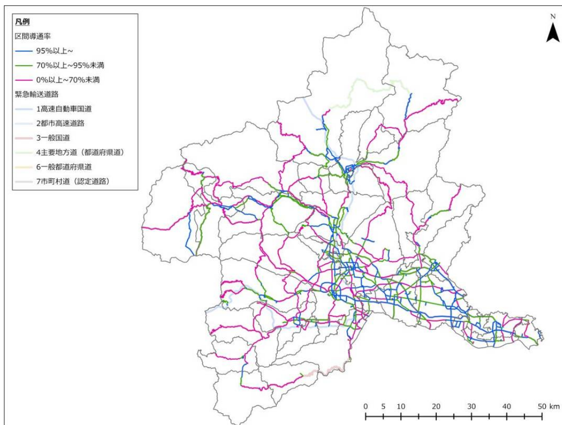
図 3-4-19 2 地点間の導通率（深谷断層帯・綾瀬川断層、冬 18 時、強風）
