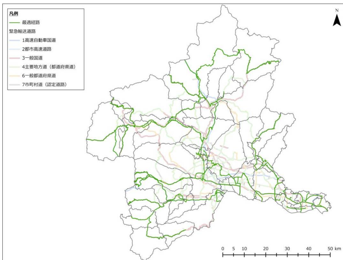
図 3-4-41 主要都市間の最適経路（太田断層、冬 5 時、強風）
