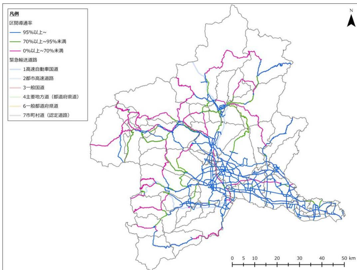
図 3-4-34 2 地点間の導通率（長野盆地西縁断層帯、冬 18 時、強風）
