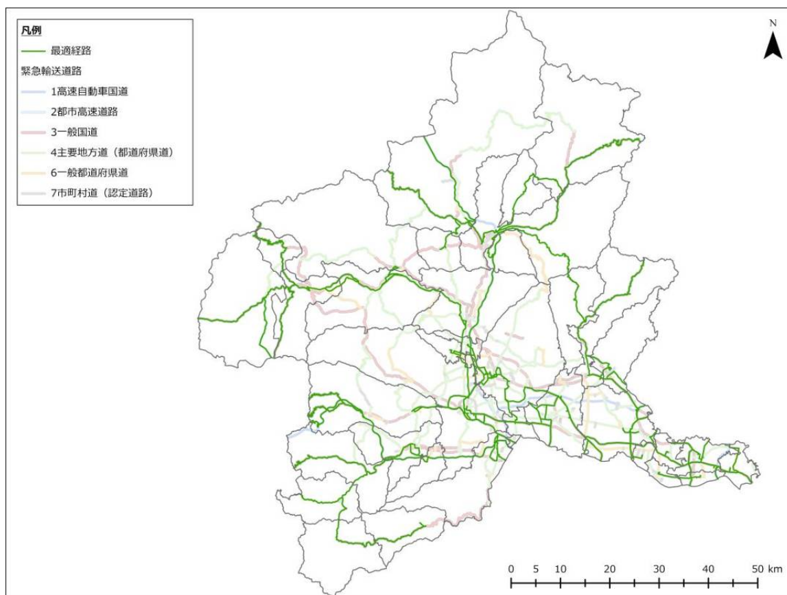
図 3-4-46 主要都市間の最適経路（大久保断層、冬 18 時、強風）
