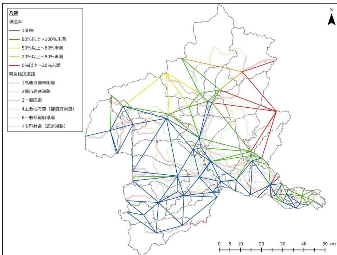
図 3-4-61 主要都市間の導通率（片品川左岸断層、冬 18 時、強風）
