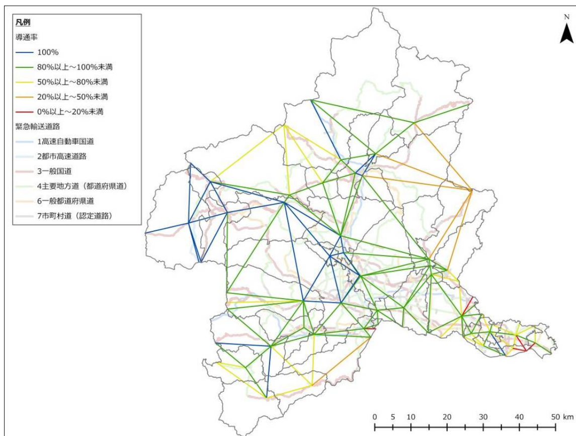
図 3-4-58 主要都市間の導通率（太田断層、冬 18 時、強風）
