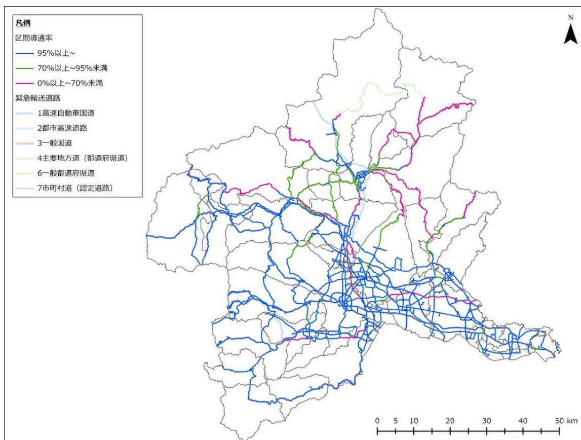
図 3-4-26 2 地点間の導通率（片品川左岸断層、冬 5 時、強風）
