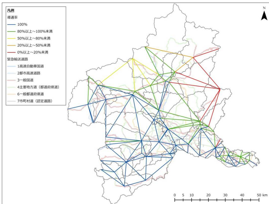
図 3-4-63 主要都市間の導通率（片品川左岸断層、夏 12 時、強風）
