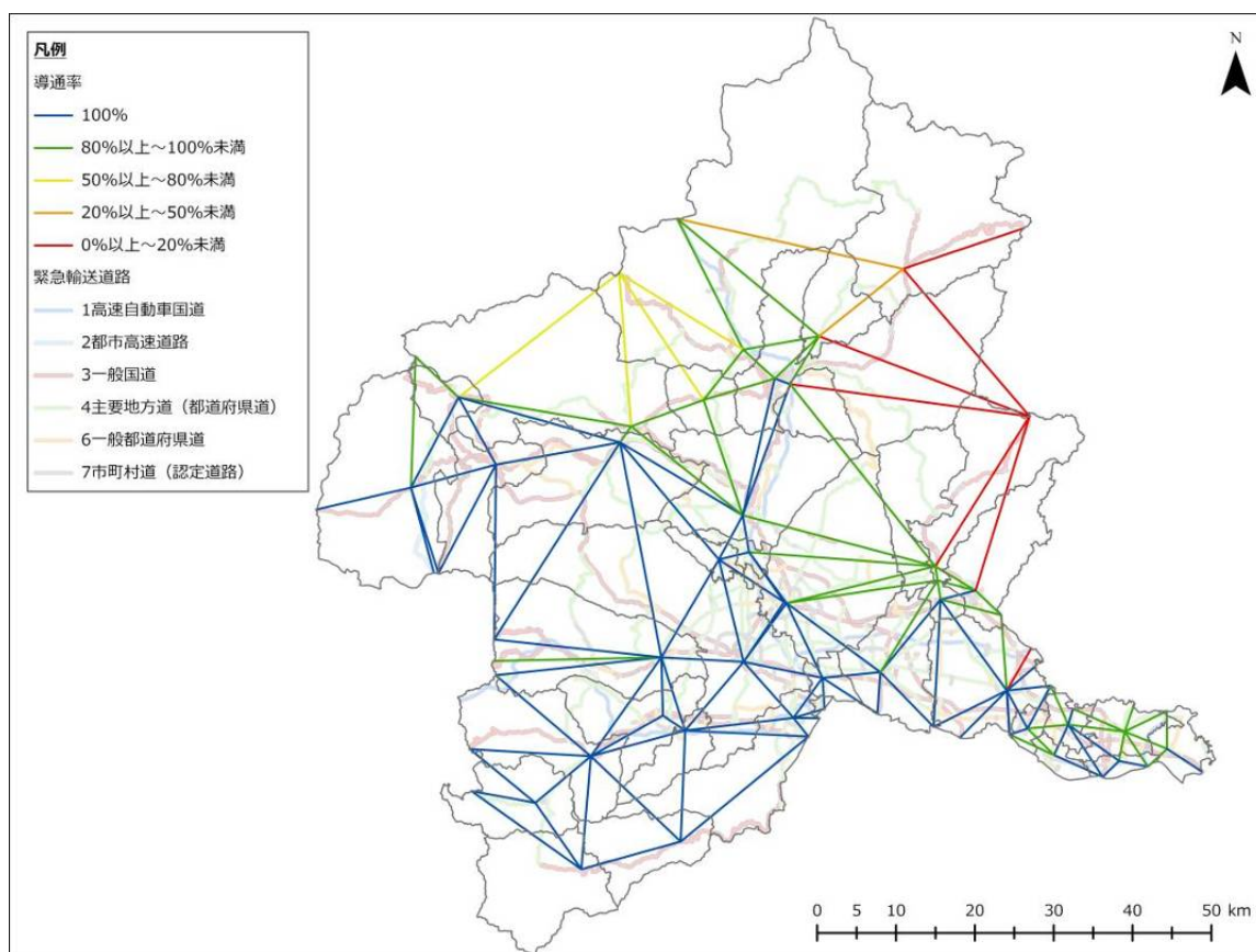
図 3-4-62 主要都市間の導通率（片品川左岸断層、冬 5 時、強風）
