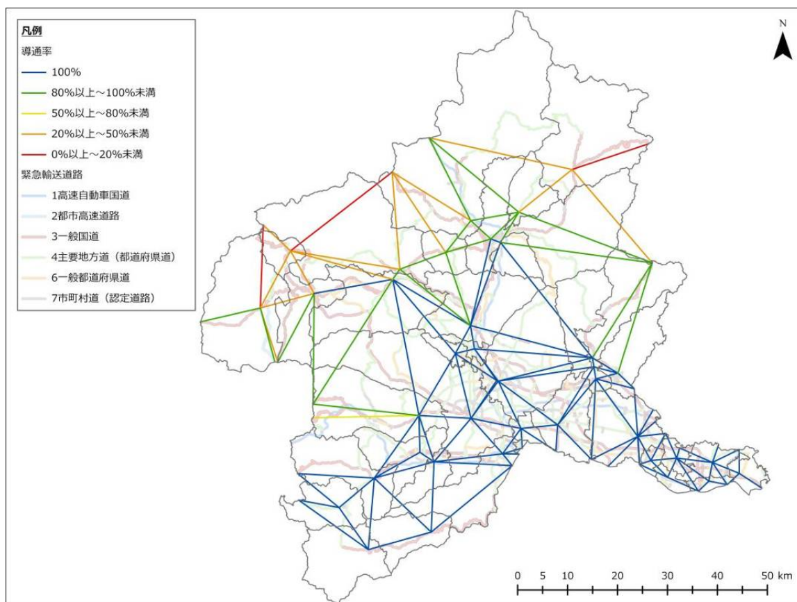
図 3-4-67 主要都市間の導通率（六日町断層帯、冬 18 時、強風）
