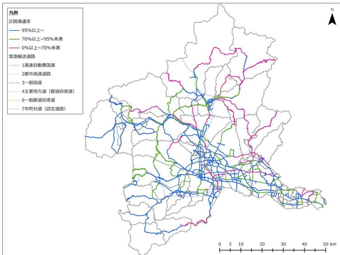
図 3-4-30 2 地点間の導通率（大久保断層、夏 12 時、強風）
