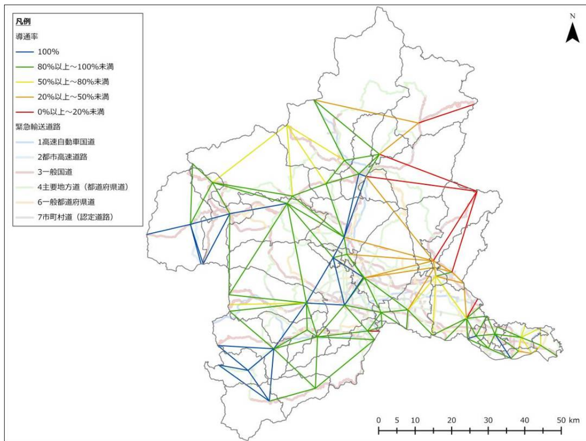
図 3-4-66 主要都市間の導通率（大久保断層、夏 12 時、強風）
