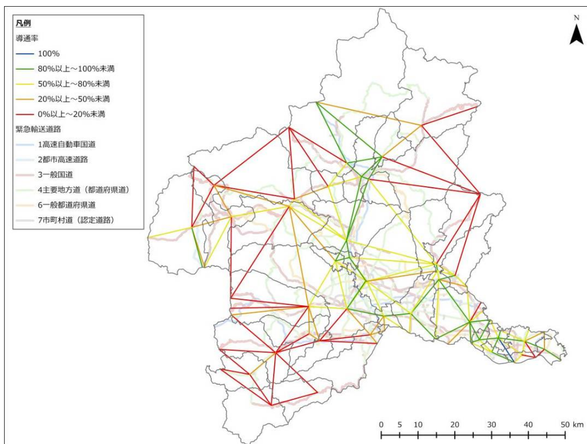
図 3-4-56 主要都市間の導通率（深谷断層帯・綾瀬川断層、冬 5 時、強風）
