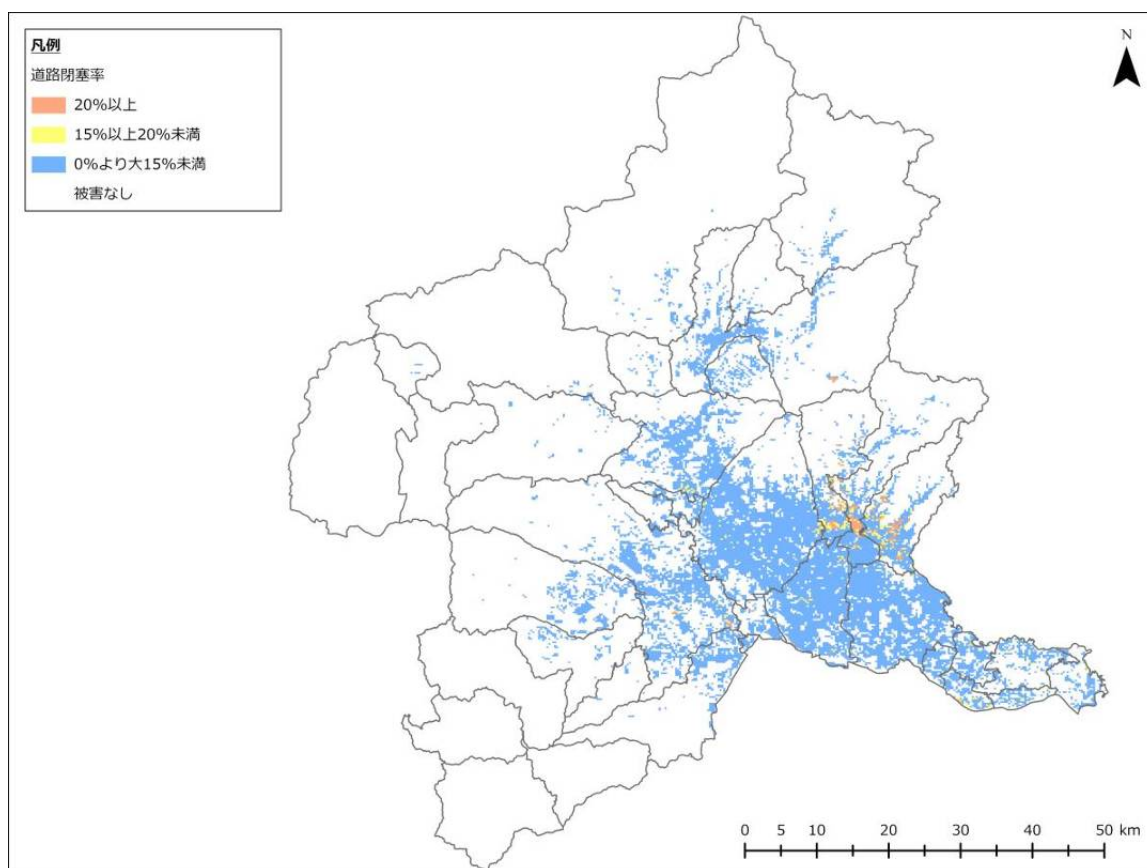
図 3-4-11 道路閉塞率（大久保断層、冬 5 時、強風）
