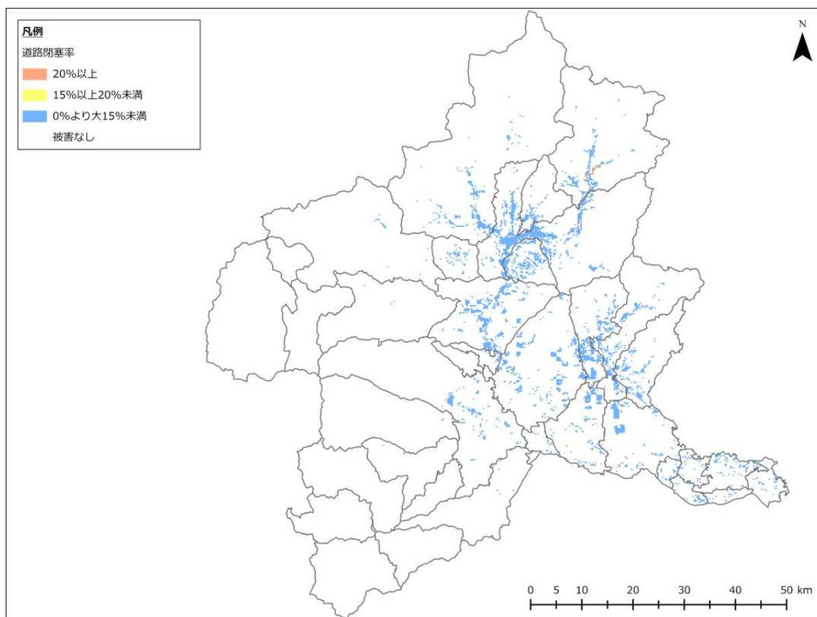
図 3-4-7 道路閉塞率（片品川左岸断層、冬 18 時、強風）
