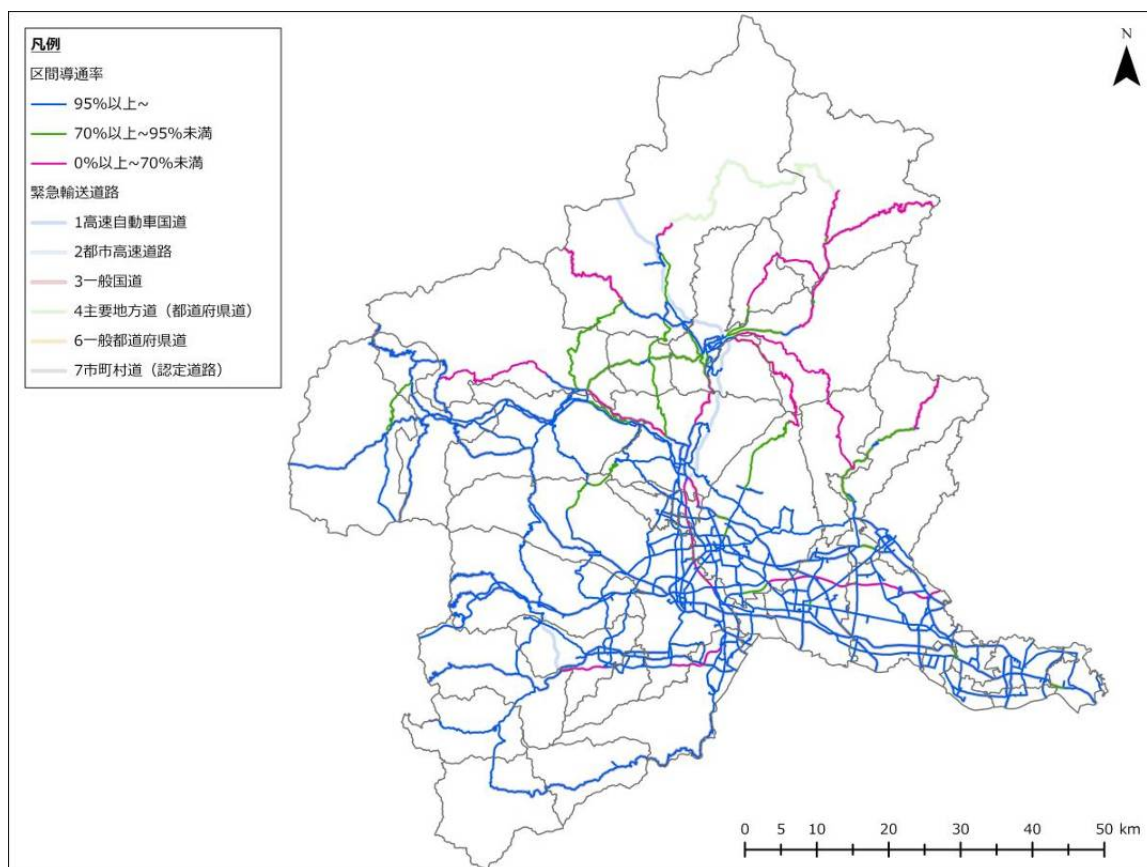
図 3-4-25 2 地点間の導通率（片品川左岸断層、冬 18 時、強風）
