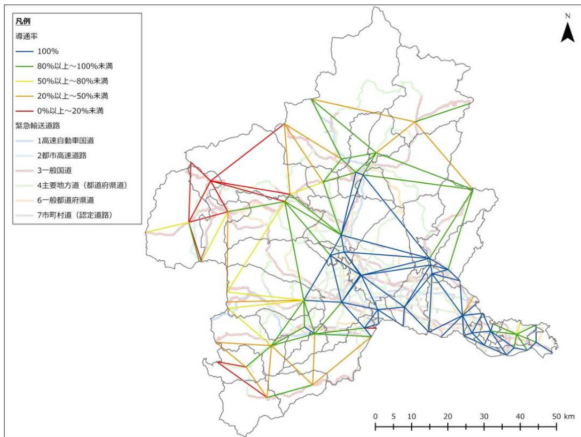
図 3-4-72 主要都市間の導通率（長野盆地西縁断層帯、夏 12 時、強風）
