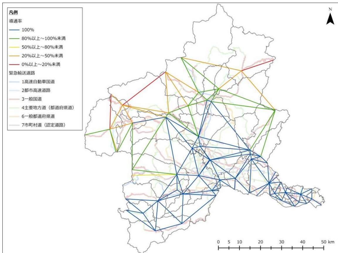
図 3-4-69 主要都市間の導通率（六日町断層帯、夏 12 時、強風）
