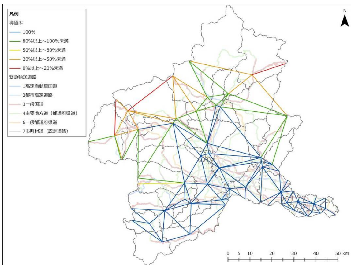
図 3-4-68 主要都市間の導通率（六日町断層帯、冬 5 時、強風）
