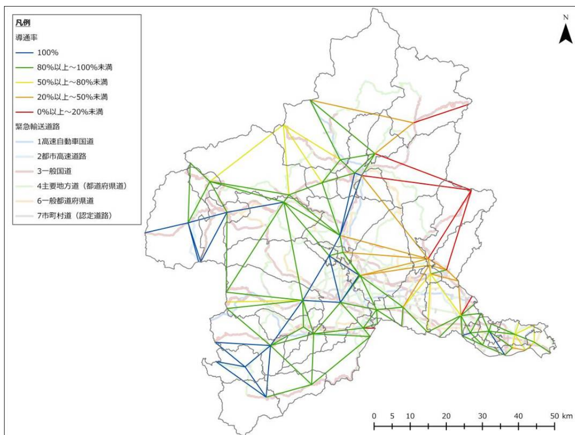
図 3-4-65 主要都市間の導通率（大久保断層、冬 5 時、強風）
