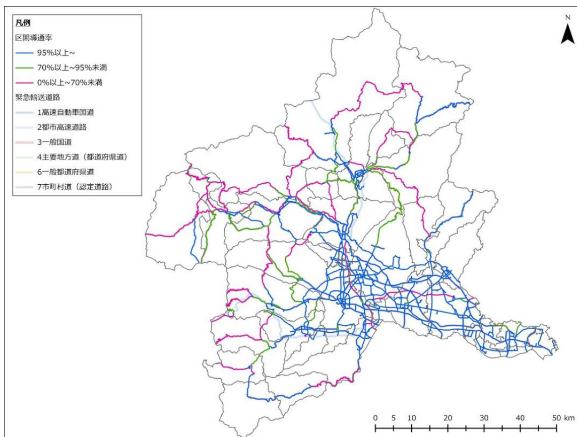
図 3-4-35 2 地点間の導通率（長野盆地西縁断層帯、冬 5 時、強風）
