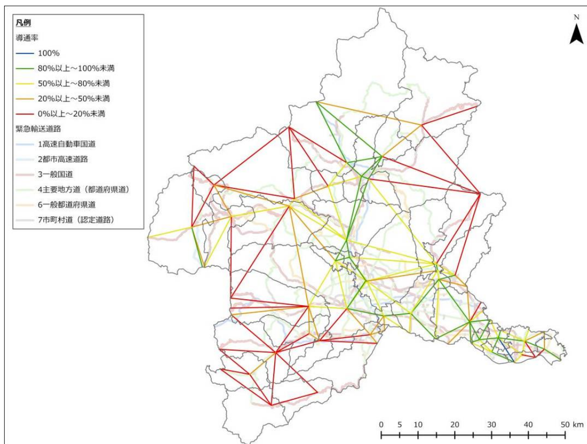
図 3-4-55 主要都市間の導通率（深谷断層帯・綾瀬川断層、冬 18 時、強風）
