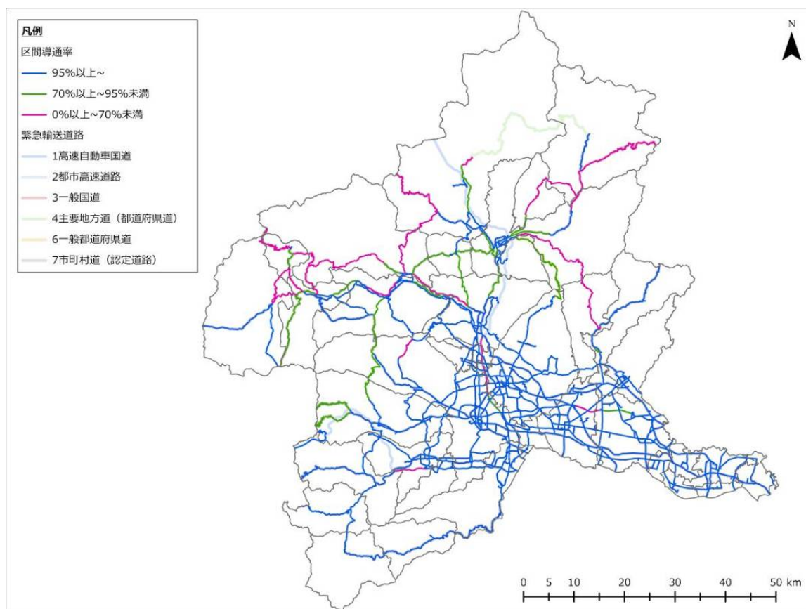
図 3-4-33 2 地点間の導通率（六日町断層帯、夏 12 時、強風）
