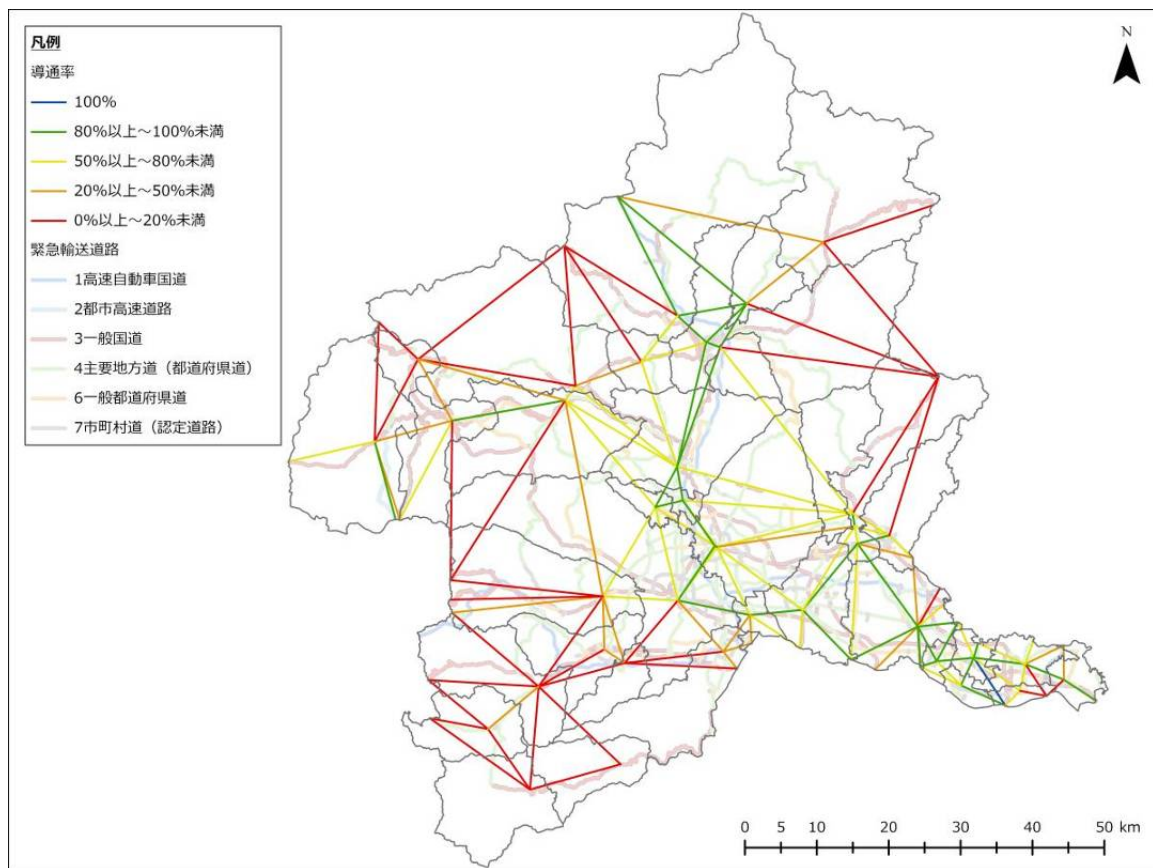
図 3-4-57 主要都市間の導通率（深谷断層帯・綾瀬川断層、夏 12 時、強風）
