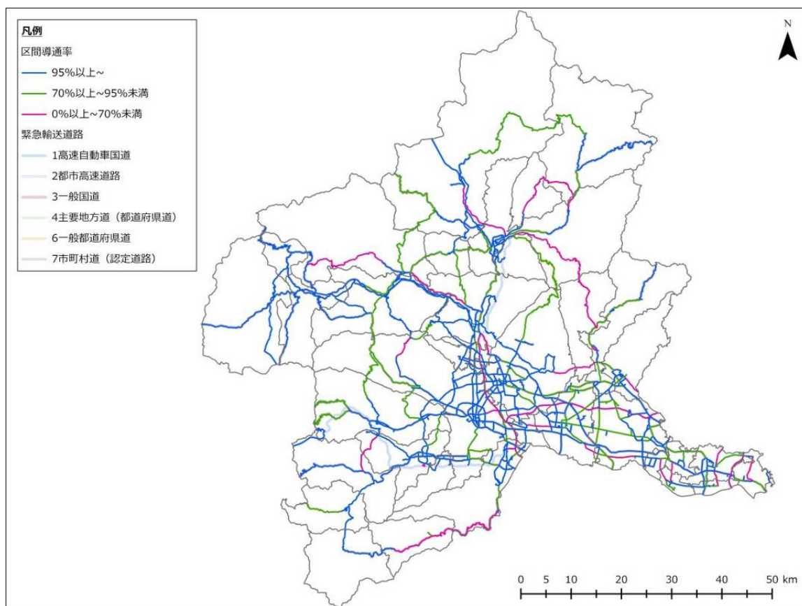
図 3-4-24 2 地点間の導通率（太田断層、夏 12 時、強風）
