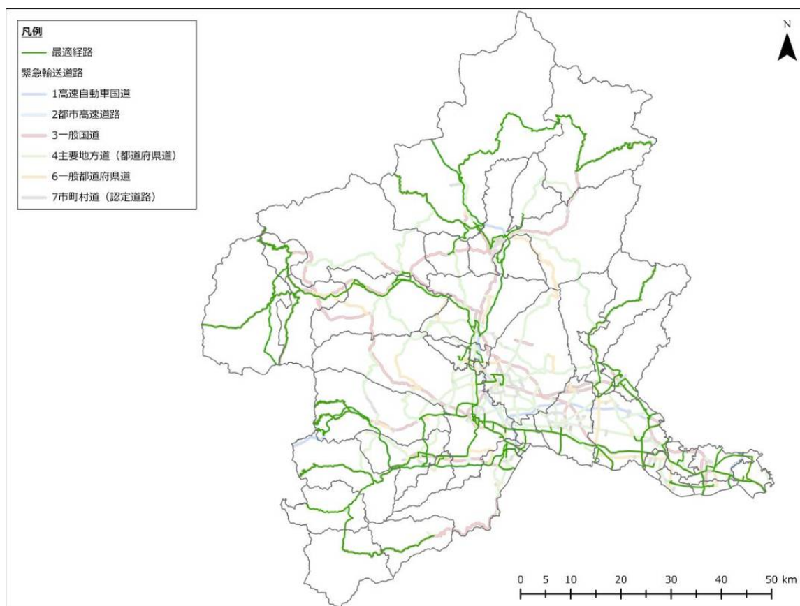
図 3-4-38 主要都市間の最適経路（深谷断層帯・綾瀬川断層、冬 5 時、強風）
