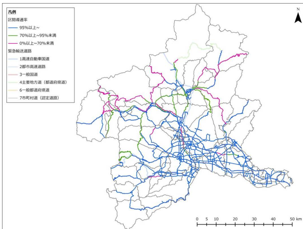
図 3-4-32 2 地点間の導通率（六日町断層帯、冬 5 時、強風）
