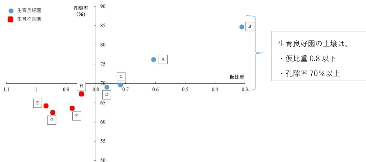
図 ブルーベリー園地の仮比重と孔隙率が生育状況に及ぼす影響
