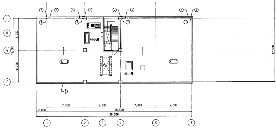
PH階平面図
