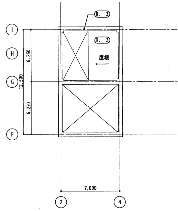
PHR階平面図
