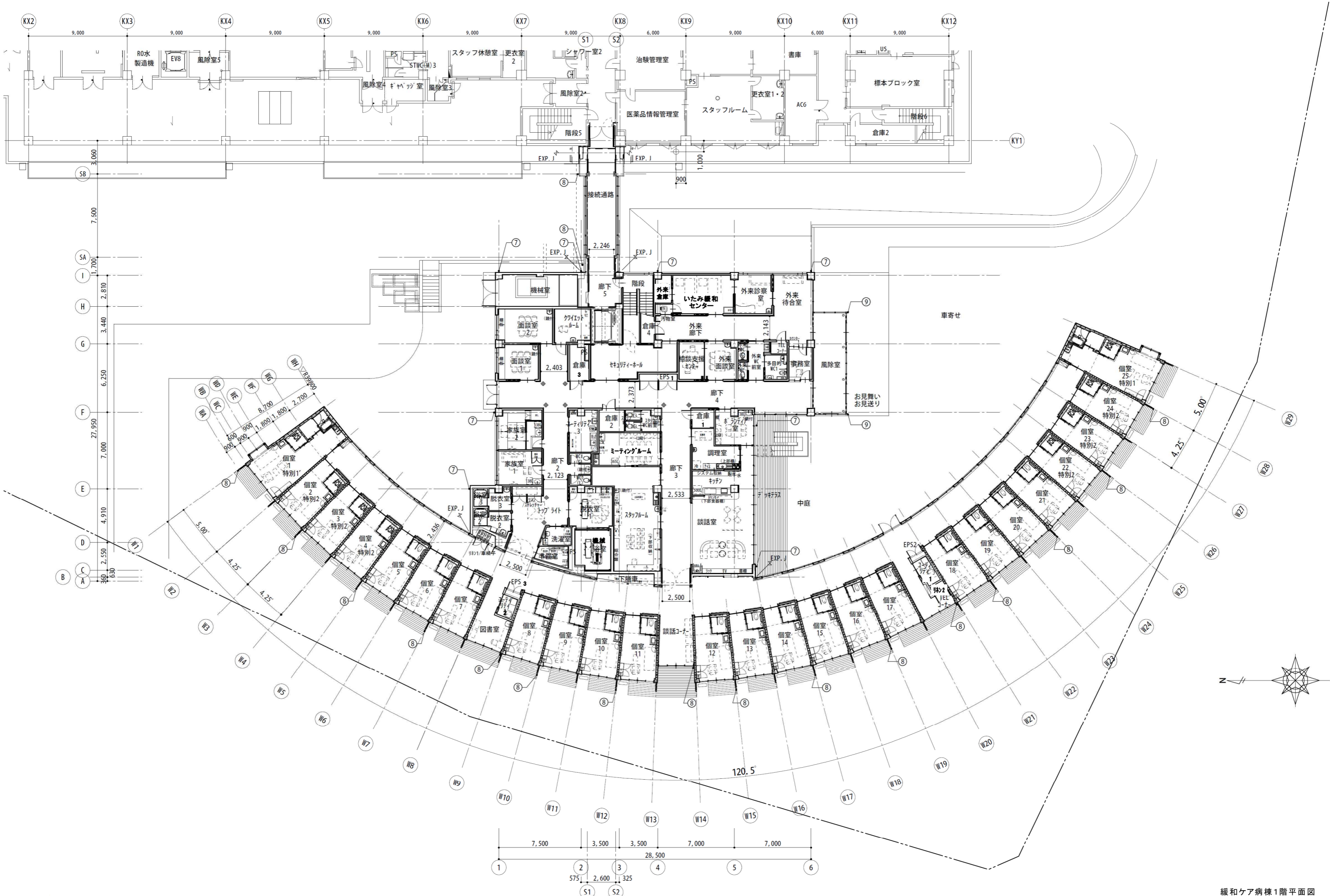
緩和ケア病棟1階平面図
