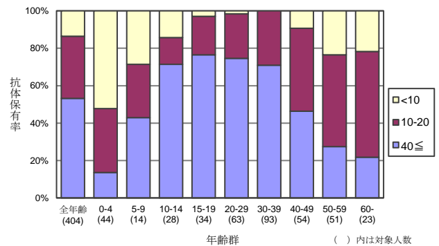
図 4 年齢群別インフルエンザ HI 抗体保有状況 A/香港/2671/2019 (H3N2)
