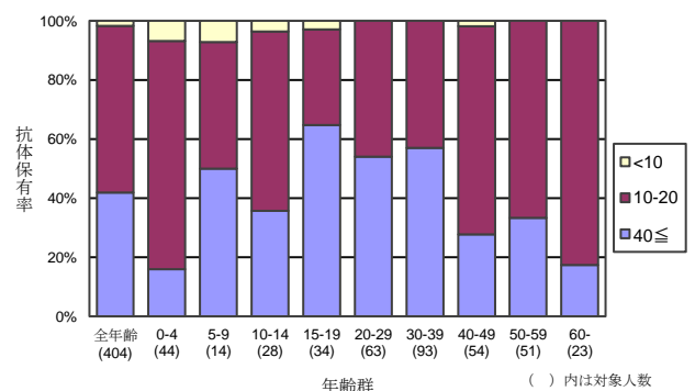
図 6 年齢群別インフルエンザ HI 抗体保有状況 B/プーケット/3073/2013 (山形系統)
