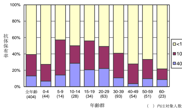
図 3 年齢群別インフルエンザ HI 抗体保有状況 A/広東-茂南/SWL1536/2019 (H1N1)
