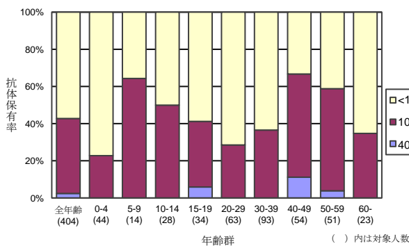
図 5 年齢群別インフルエンザ HI 抗体保有状況 B/ビクトリア/705/2018 (ビクトリア系統)
