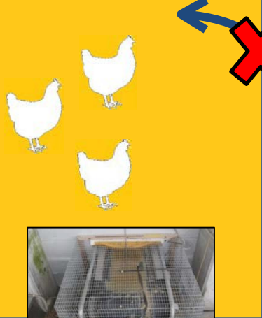
集卵・除糞ベルトの開口部の隙間対策
