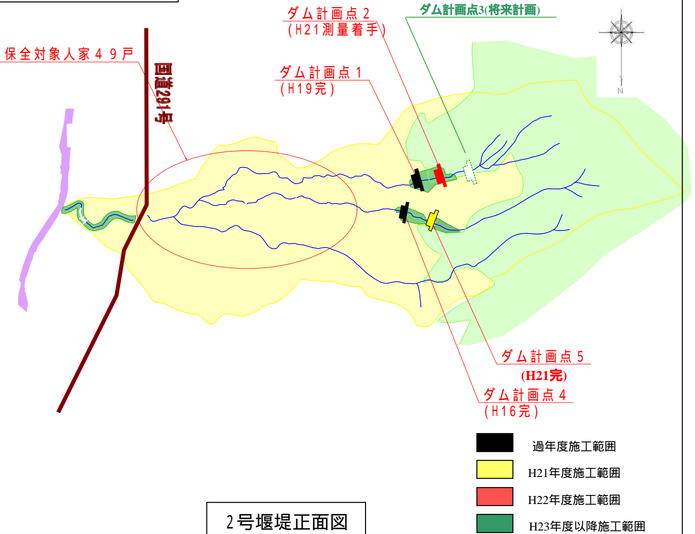
流域概要図
