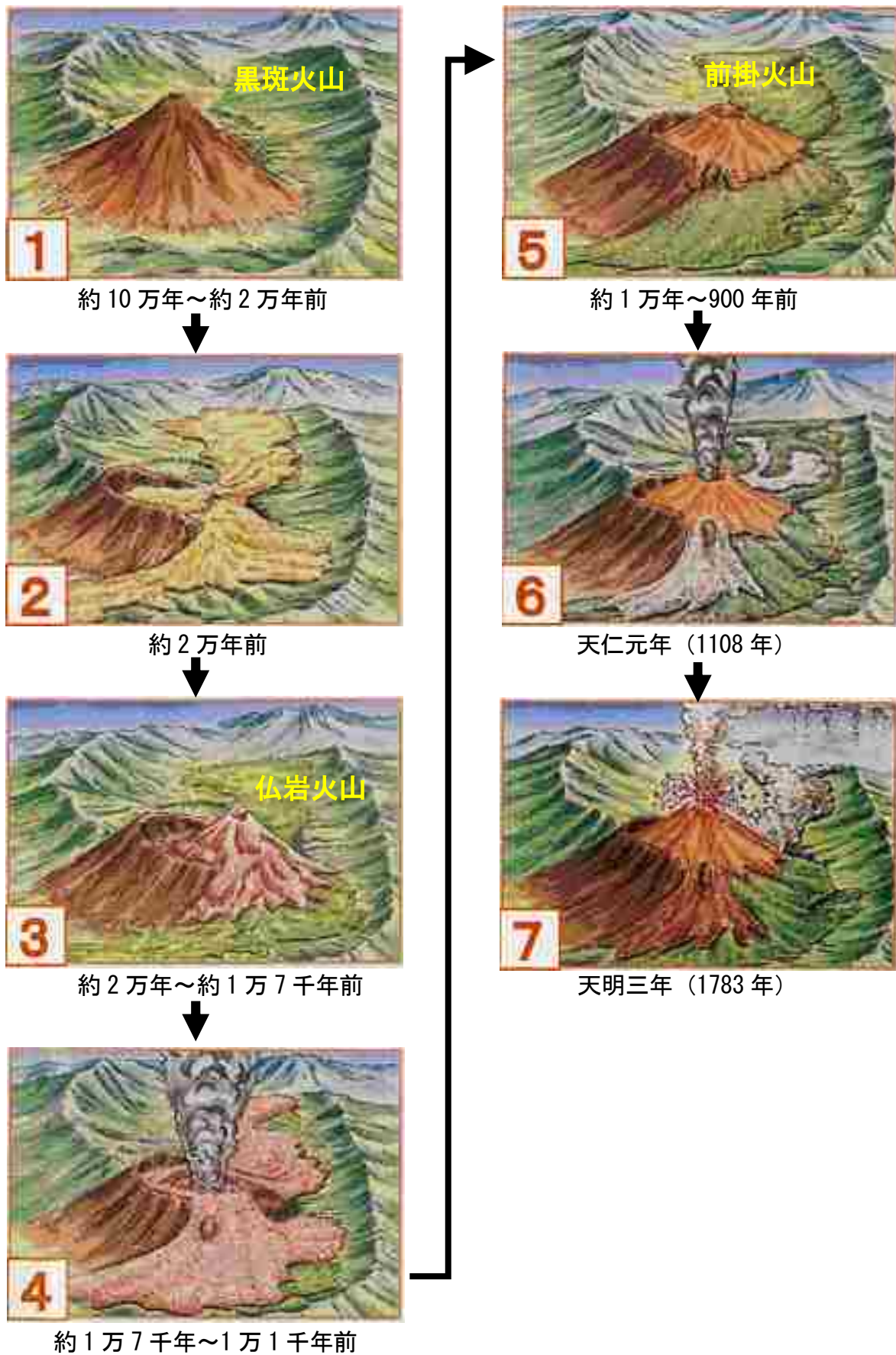
図一2.1.2 浅間山の形成史
