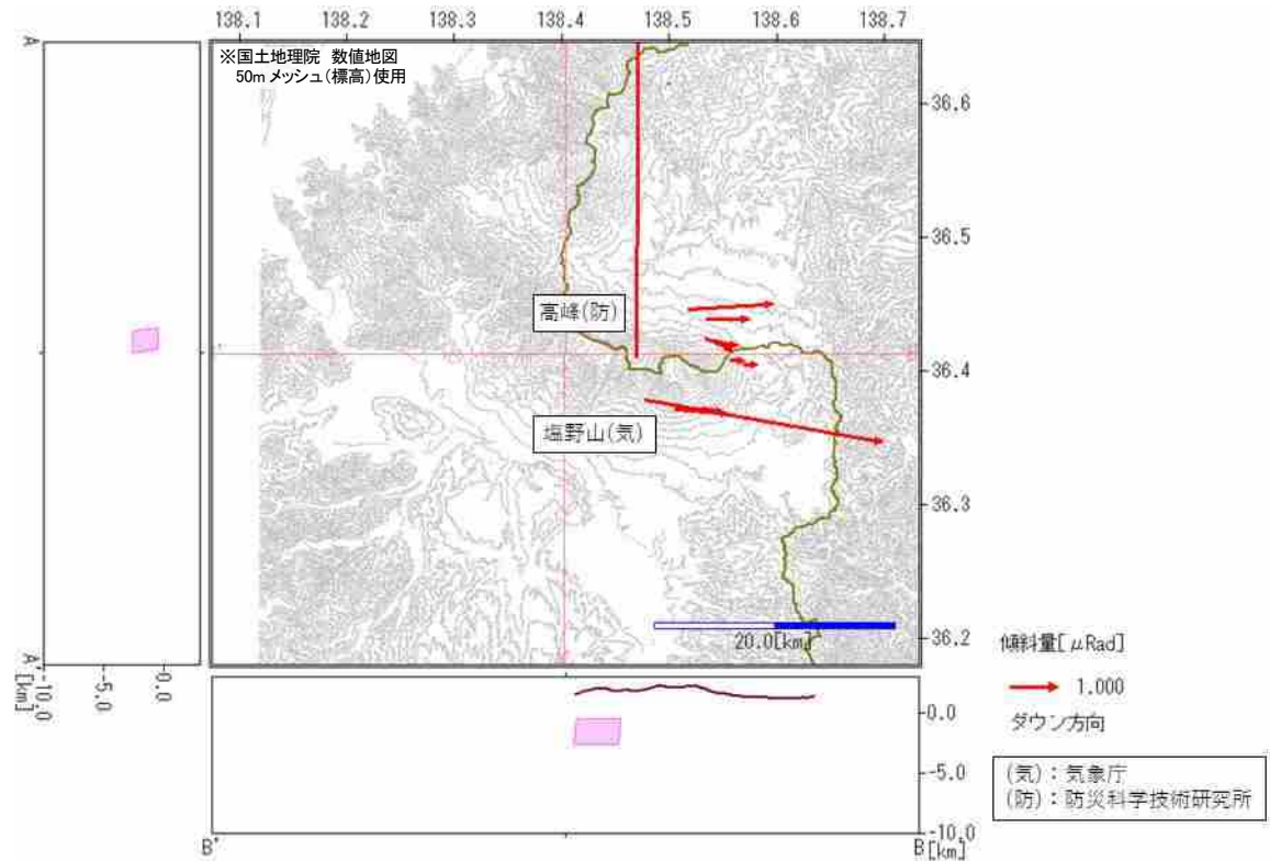
参考図-4 山体西麓への急激なダイク貫入を示す傾斜変化の予測量の一例 (浅間山西麓の深さ 1.5km (海面下) の場所に、体積変化量 0.01\text{km}^3 のマグマがダイク状に貫入 (体積膨張) すると仮定した場合の推定変動量)
