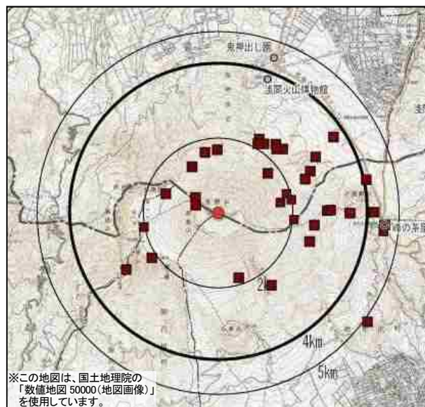
図-3.1.3 直径20～30cmの噴石分布 (1920年～2004年)
