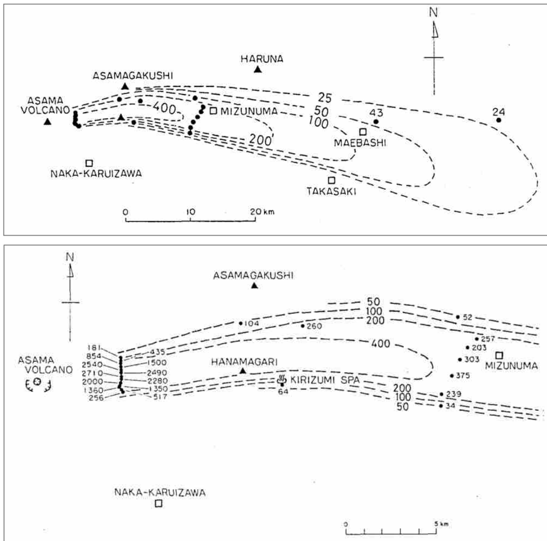
図-3.1.4 1983年4月8日の噴火の降灰量分布図 [g/m 2 ] 荒牧ほか(1983) 24 より
