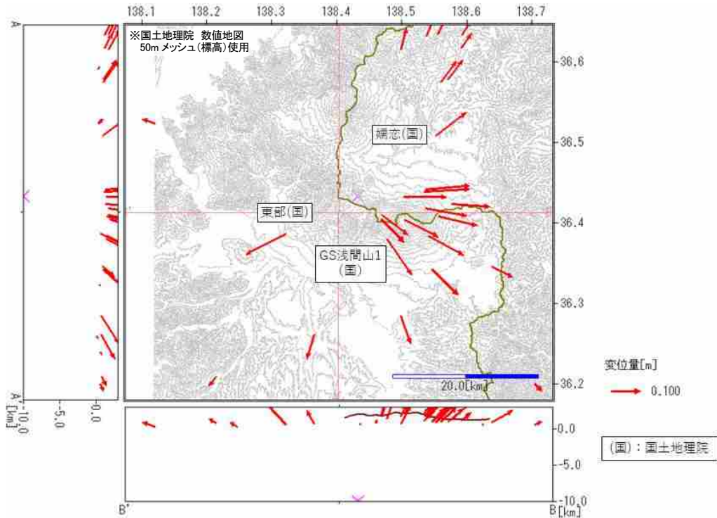
参考図-1 深部マグマ溜りへのマグマ蓄積を示す地殻変動 (GNSS) の予測量の一例 (深部マグマ溜りの深さを10kmと仮定し、天明噴火及び天仁噴火の総マグマ噴出量を参考に、 深部マグマ溜りに0.22km 3 のマグマが蓄積(球状に膨張)すると仮定した場合の推定変動量)
