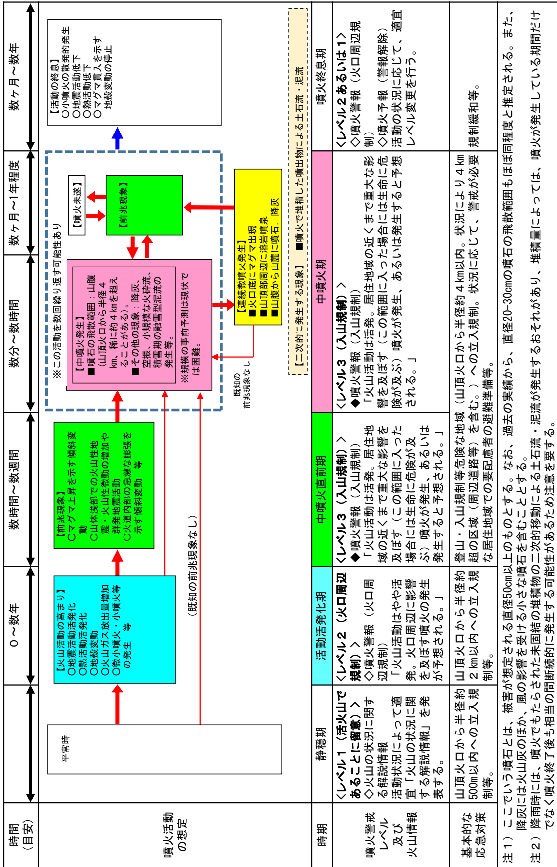
図2の2 浅間山のシナリオフロー図 (中噴火のケース)
