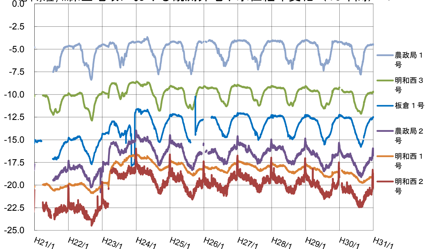
地下水水位 / m 保全地域における観測井地下水水位経年変化（10年間） -1
