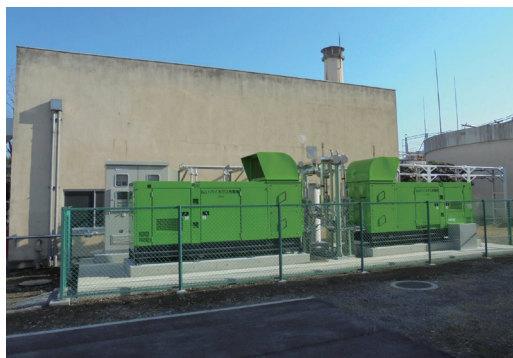
バイオマス発電(伊勢崎センター(伊勢崎市))
