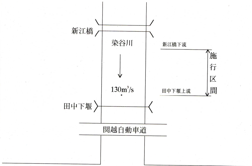
計画流量配分図
