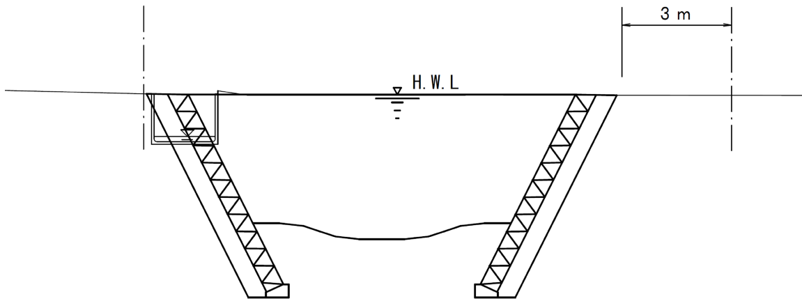
代表横断面図（市道0232号線上流地点）
