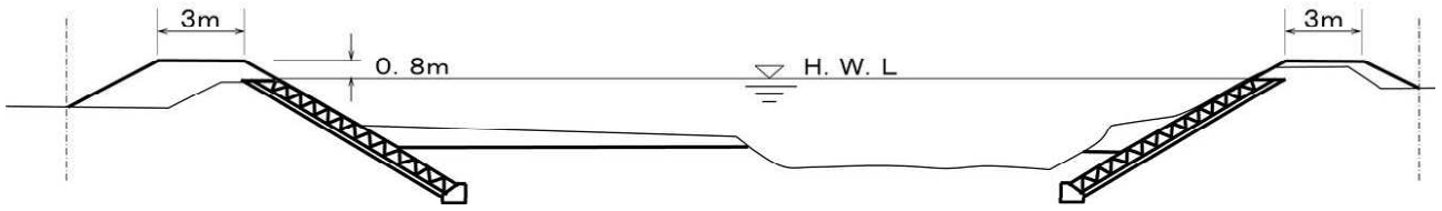
代表横断面図（一貫堀川合流点下流付近）
