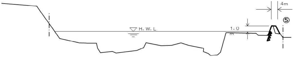
⑤代表横断面
