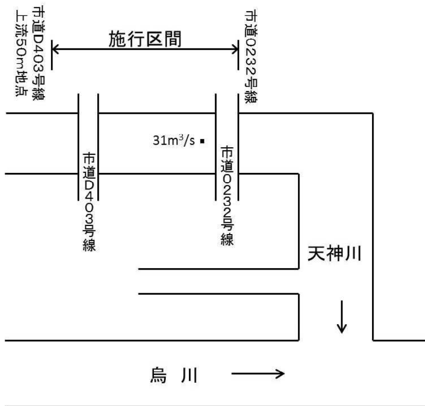
計画流量配分図
