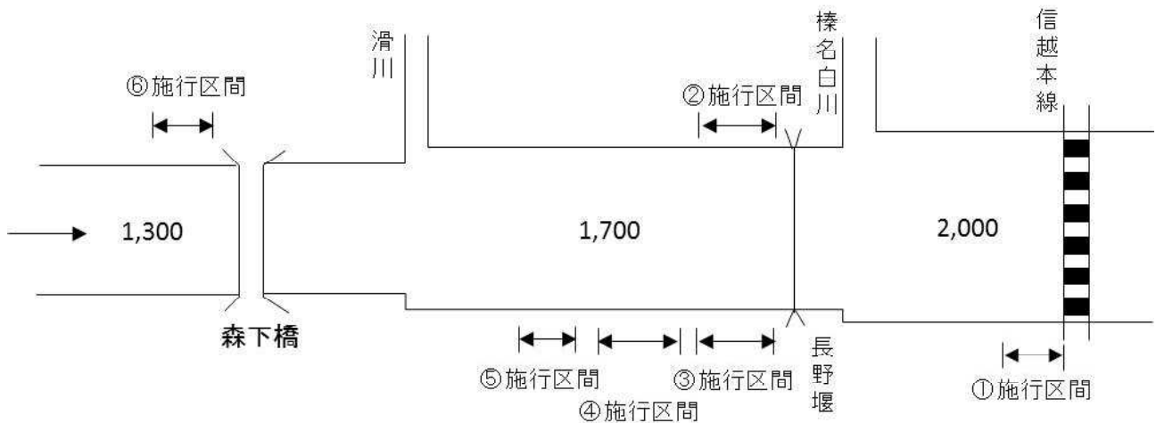
計画流量配分図
