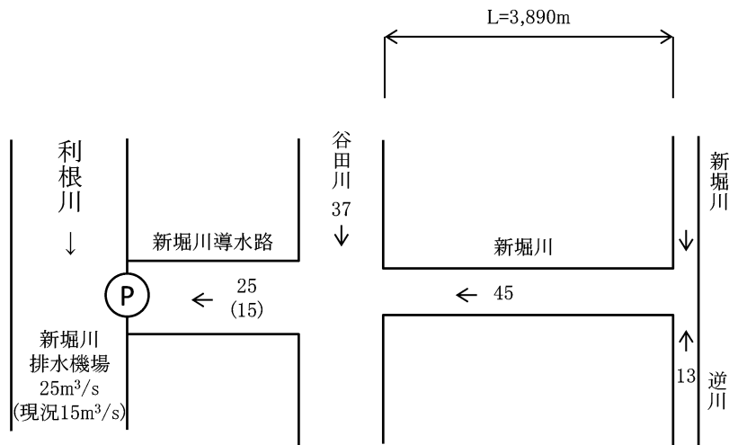
図 4.15 流量配分図(新堀川)
