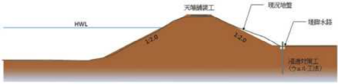
図 4.23 代表横断図(堤防強化対策)
