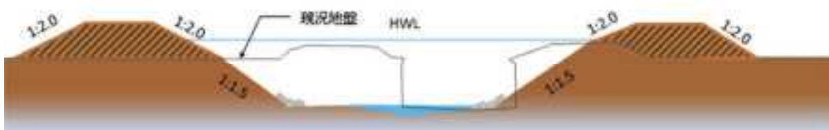
図 4.6 代表横断面図(多々良川)
