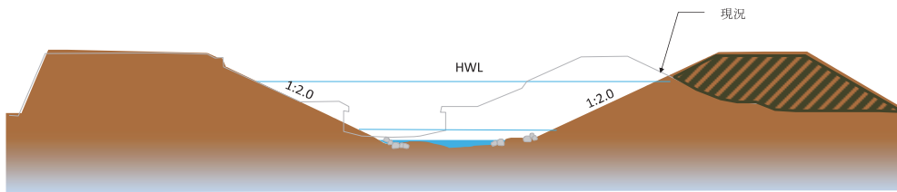
図 4.14 代表横断面図(新堀川)
