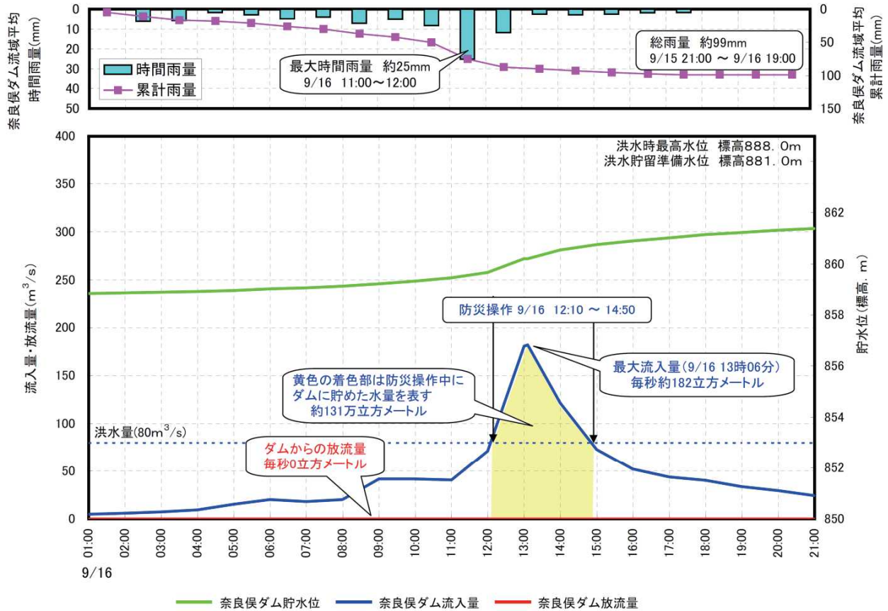
図14 ダムの防災操作の状況図
