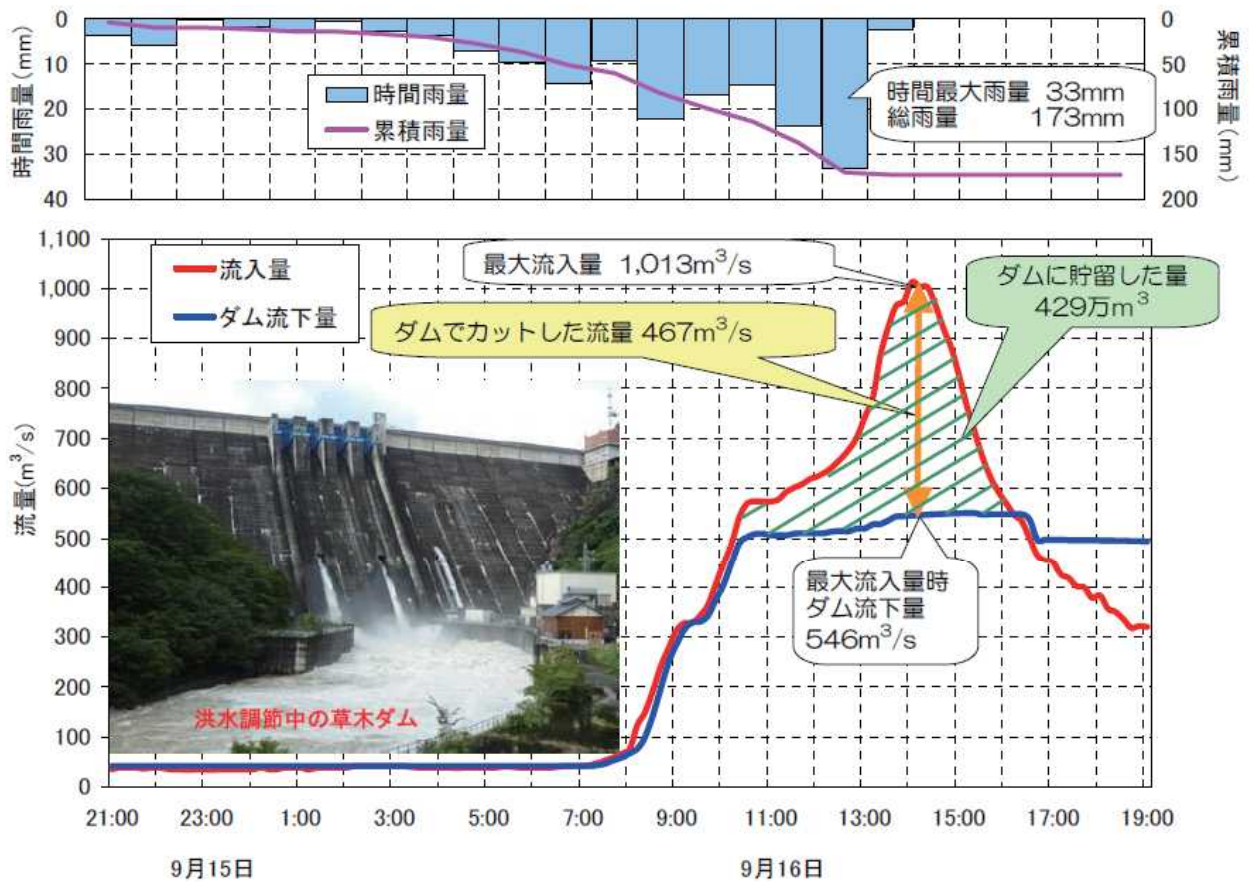
図12 ダムの効果と防災操作実績図 出典: 草木ダムにおける防災操作(洪水調節)の効果
