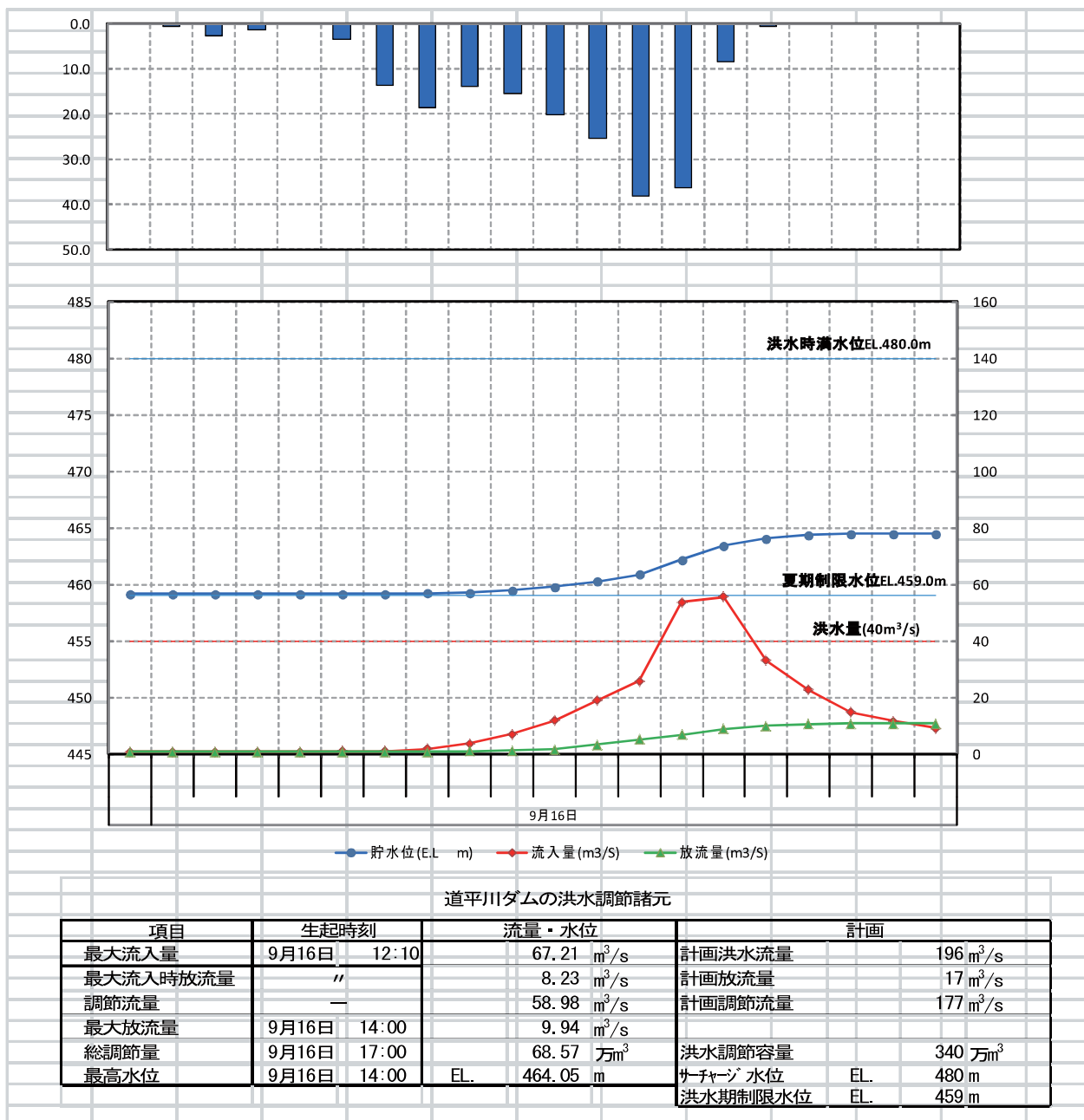
図10 ダムの調節状況と貯留状況
