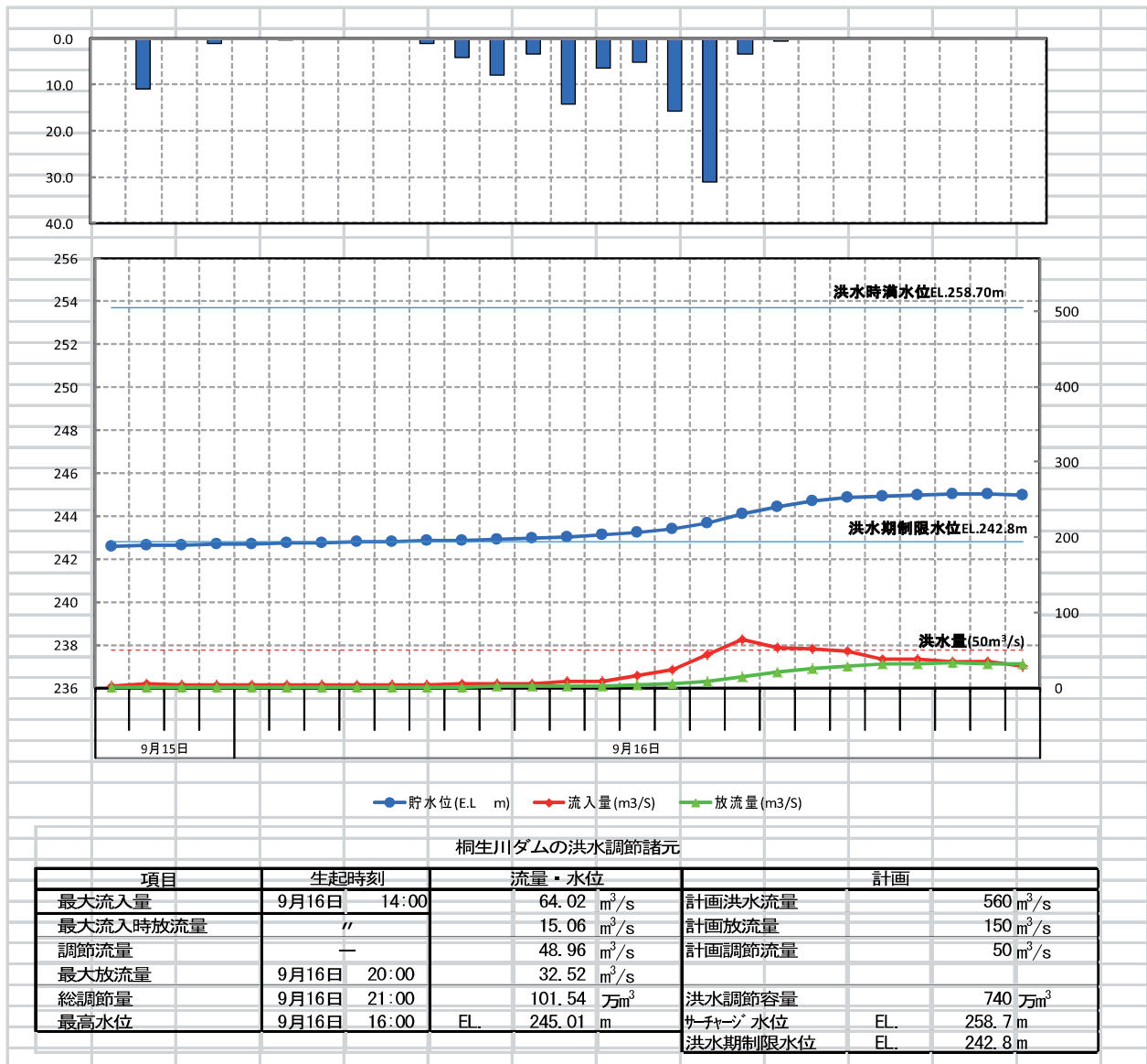
図8 ダムの調節状況と貯留状況
