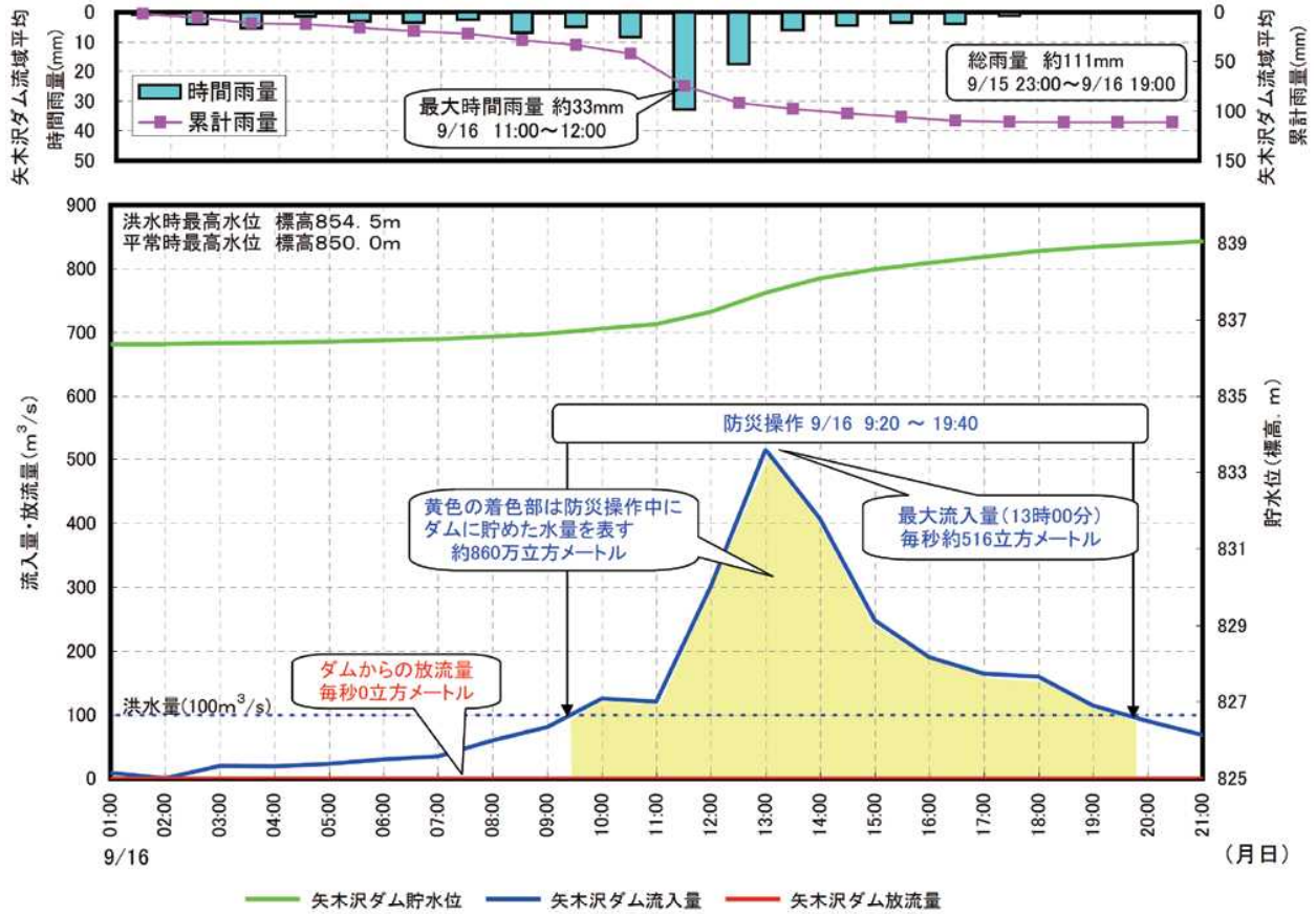
図13 ダムの防災操作の状況図
