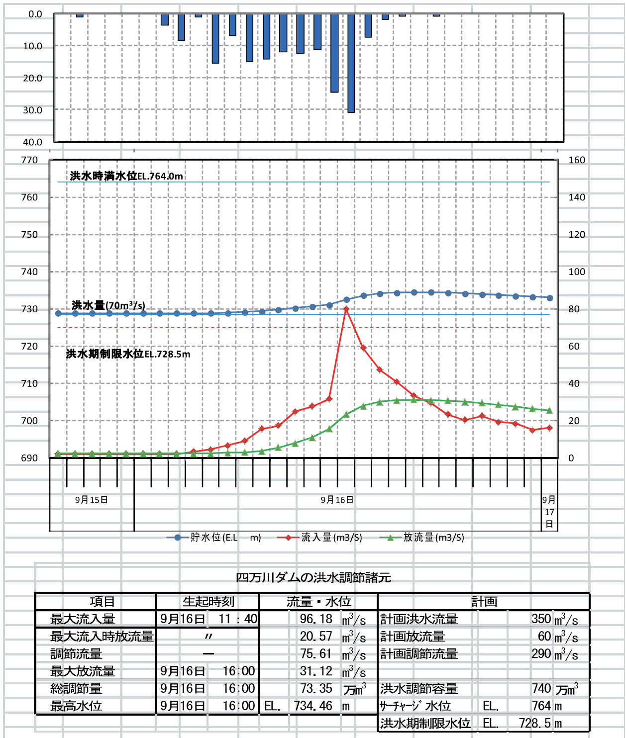
図9 ダムの調節状況と貯留状況
